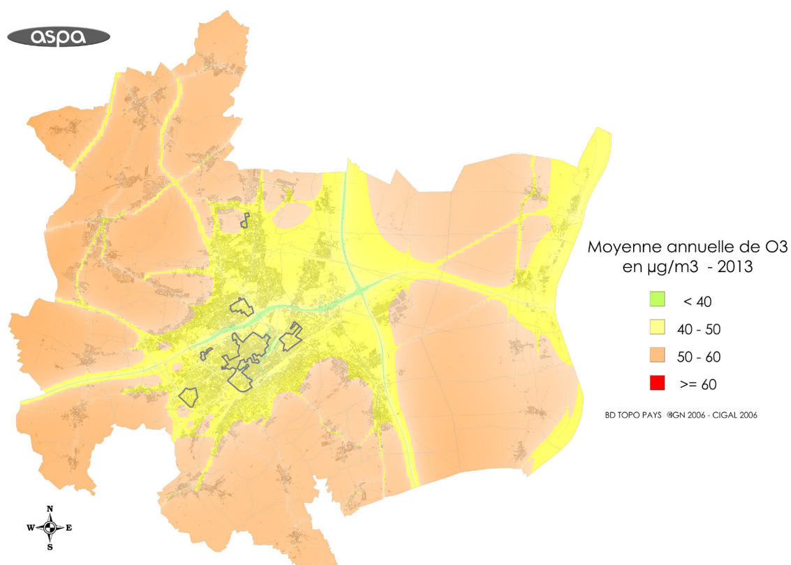
Carte 34 : Moyenne annuelle de O3 en \mu\text{g}/\text{m}^3 en 2013
