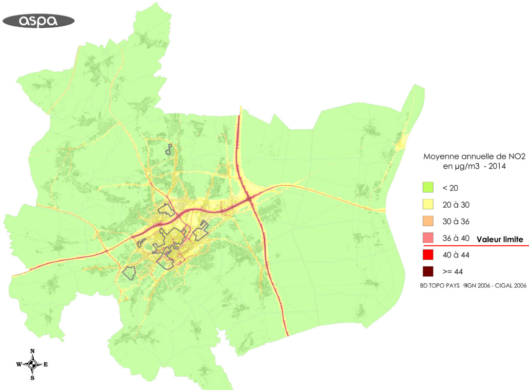
Carte 29 : Moyenne annuelle de NO 2 en µg/m 3 en 2014
