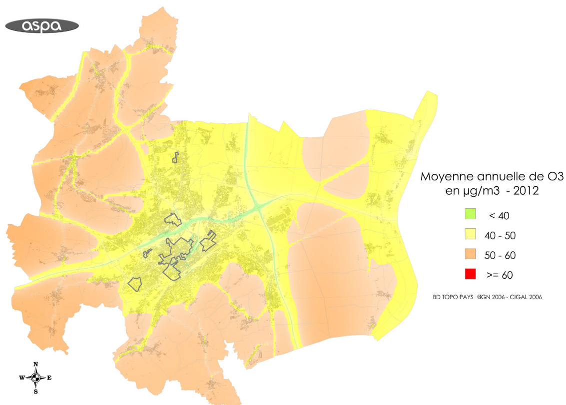
Carte 33 : Moyenne annuelle de O3 en \mu\text{g}/\text{m}^3 en 2012
